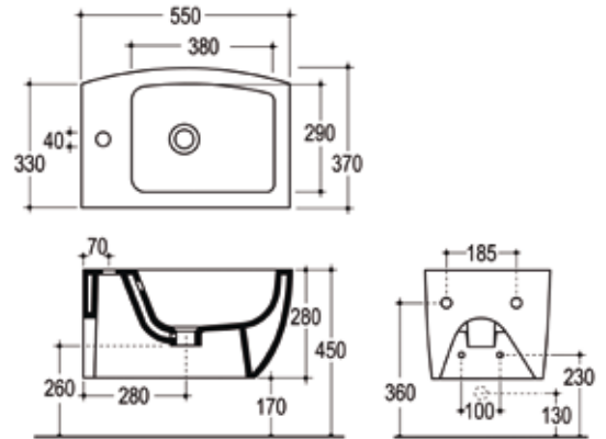
OLYBIS Bidet monoforo sospeso Wall hung single-hole bidet
