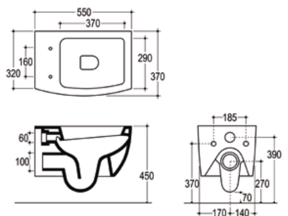
OLYVAS Vaso sospeso Wall hung WC
