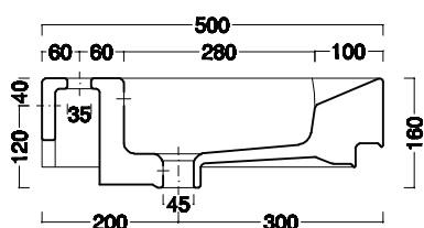
Sezione longitudinale
